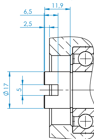
A-A 1:1
