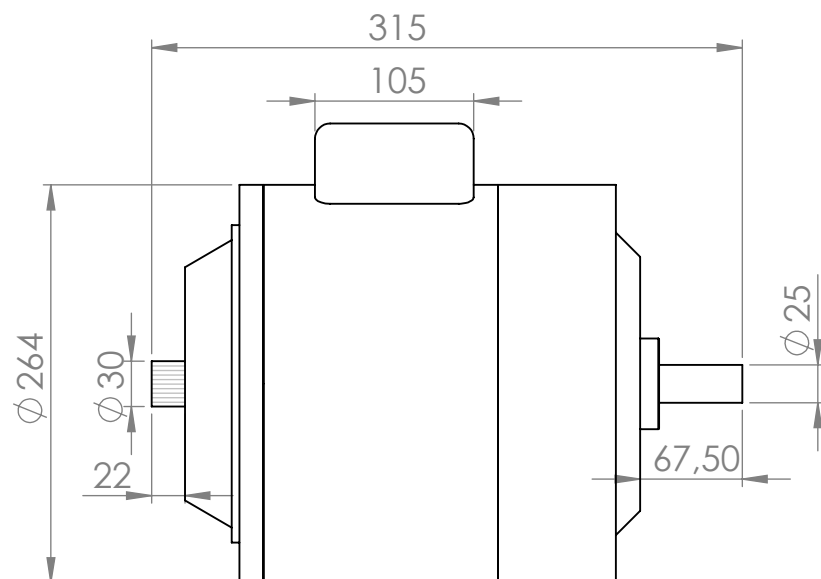
Silnik szeregowy prądu stałego
